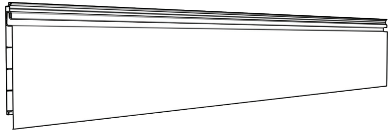
Panneau CrownWall MC de 15,24 cm (6 po) 144 cm +/- 0,6 cm (48 po +/- 1/4 po) 8 Pièces
